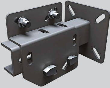
C Karkas Konsolu C Shaped Frame Bracket Кронштейн С Образной Рамы
