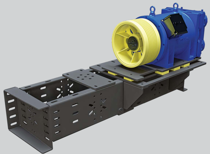
MRL Dişlisiz Tip 3 MRL Gearless Type 3 Без М.П (Безредукторная) - Тип 3
