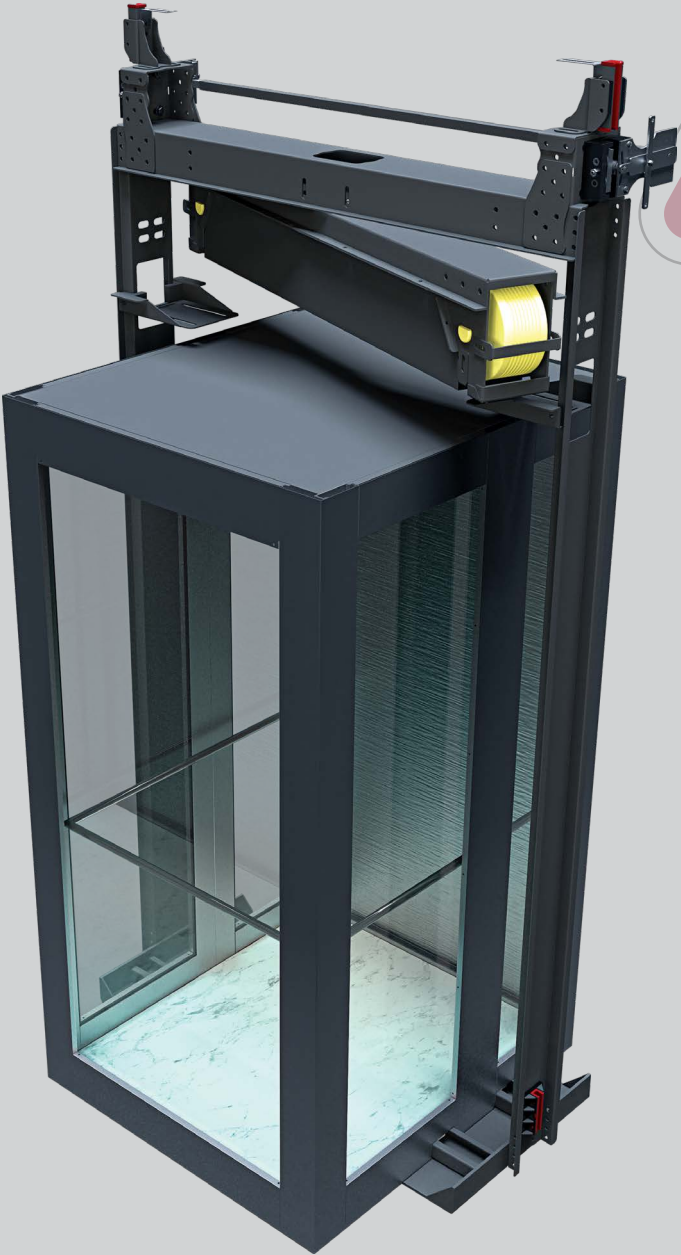
Kuyu Dibi 13 cm Pit 13 cm Прямок 13 см
