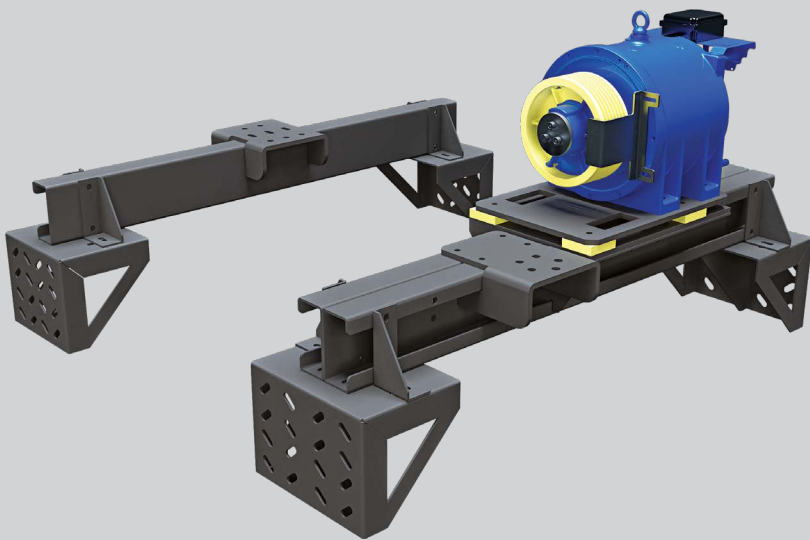
MRL Dişlisiz Tip 2 MRL Gearless Type 2 Без М.П (Безредукторная) - Тип 2
